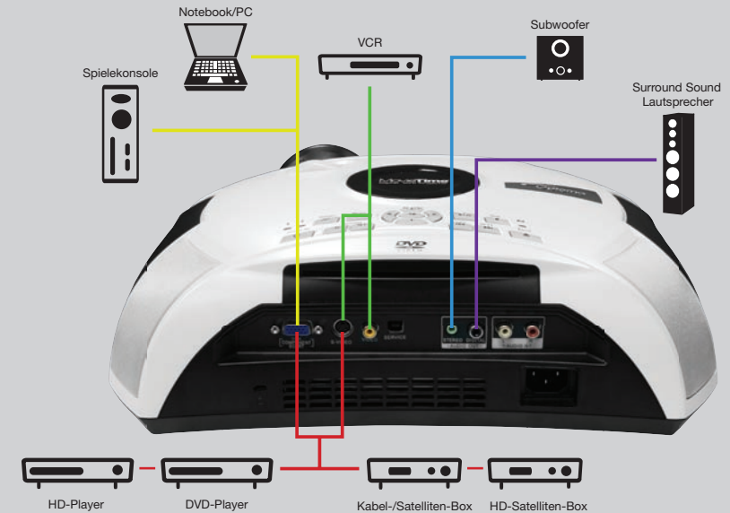
HD-Eingänge/-Bilder werden auf 480p heruntergerechnet
